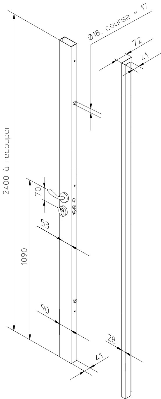
gâche standard monobloc en J
