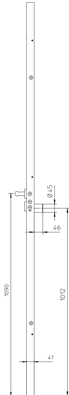
profil
